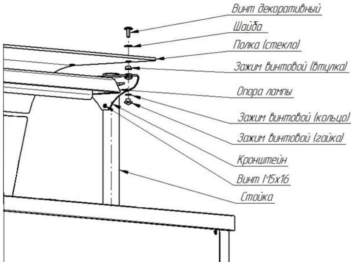
Рис.2 Сборка полок.
